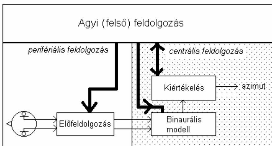
5. ábra. A hallórendszer feldolgozási lépései. A perifériális (fülek szintjén) lévő feldolgozást éppúgy felügyeli az agy, mint a centrális lépéseket, melyek során a két füljel binaurális és interaurális kiértékelése történik [42].
