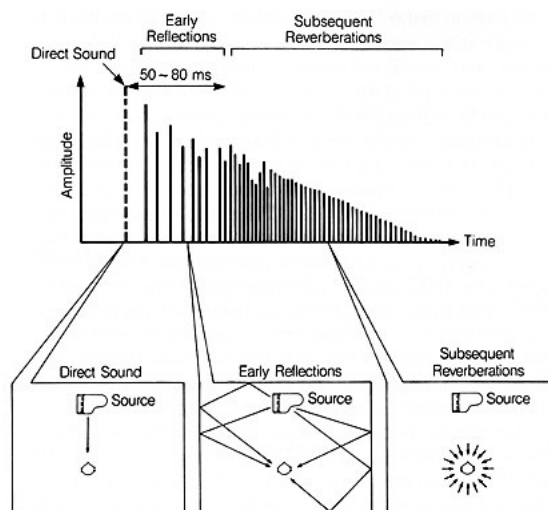
4.1 ábra Utószengés kialakulása
